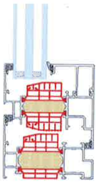
Vleugel Ouvrant
