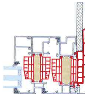
Basis profiel Profil d'appui
