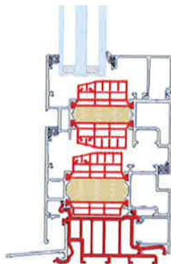
Basis profiel Profil d'appui
