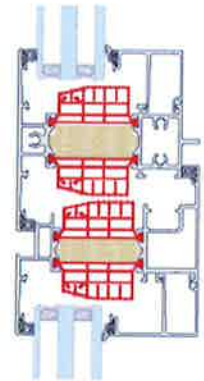
T-profiel bovenlicht Traverse imposte
